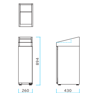
⑤⑥⑦⑧本体（投入口はタイプにより異なります。）
