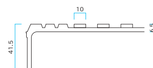
⑥⑦ステップ FS・FW
