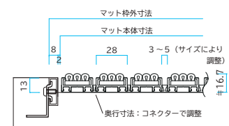
⑧Clic-19 ライト (軽歩行向け)
