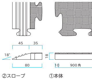
①本体・ピンク
